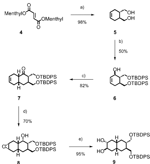
Scheme 2. Enantioselective synthesis of decalin 9 : a) i) 1,3-butadiene, \text{Et}_2\text{AlCl} , toluene, -78 \rightarrow 20^\circ\text{C} ; ii) \text{LiAlH}_4 , THF; b) i) TBDPSCl, imidazole, \text{CH}_2\text{Cl}_2 ; ii) \text{SeO}_2 , dioxane/water; c) i) \text{MnO}_2 , \text{CH}_2\text{Cl}_2 ; ii) 1,3-butadiene, \text{AlCl}_3/\text{AlMe}_3 , toluene, -78 \rightarrow 20^\circ\text{C} ; d) i) \text{NaBH}_4 , \text{CH}_2\text{Cl}_2/\text{MeOH} ; ii) m CPBA, \text{CH}_2\text{Cl}_2 , -30 \rightarrow 20^\circ\text{C} , \alpha/\beta = 9:1 ; e) i) n BuLi, PhOCSCl; ii) n Bu 3 SnH, AIBN; iii) \text{HClO}_4 , acetone.
